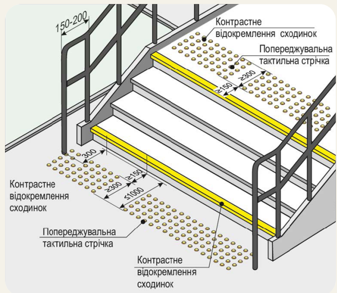
Рисунок 1.14. Облаштування сходинки
