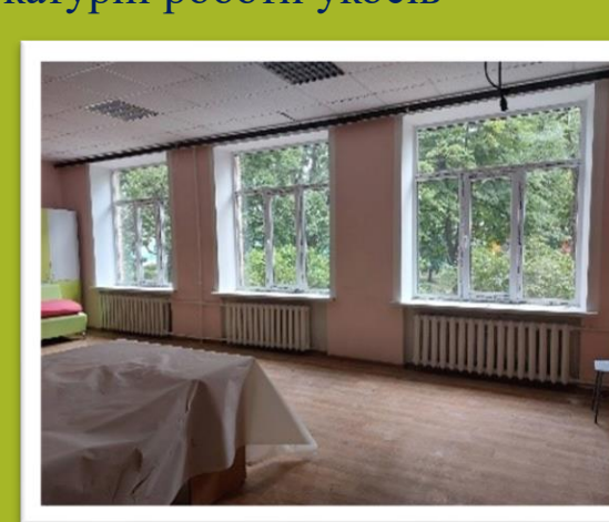
СЗШ № 4, Ліцей № 14 та СШ № 26. Встановлення нових металопластикових вікон, штукатурні роботи укосів
