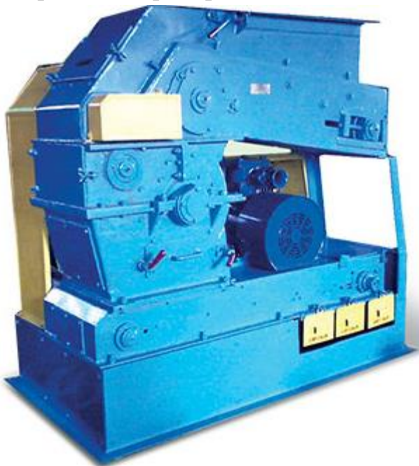
Рис. 17.2 - Проборозділювальна машина МПЛ 150М2
