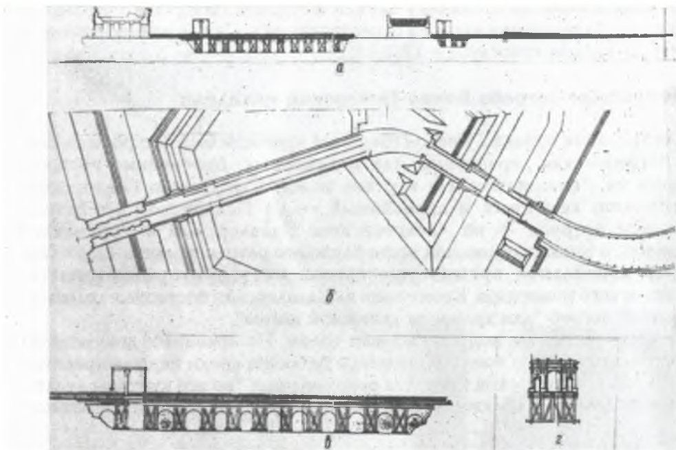
Деталі креслень головних воріт Печерської фортеці
